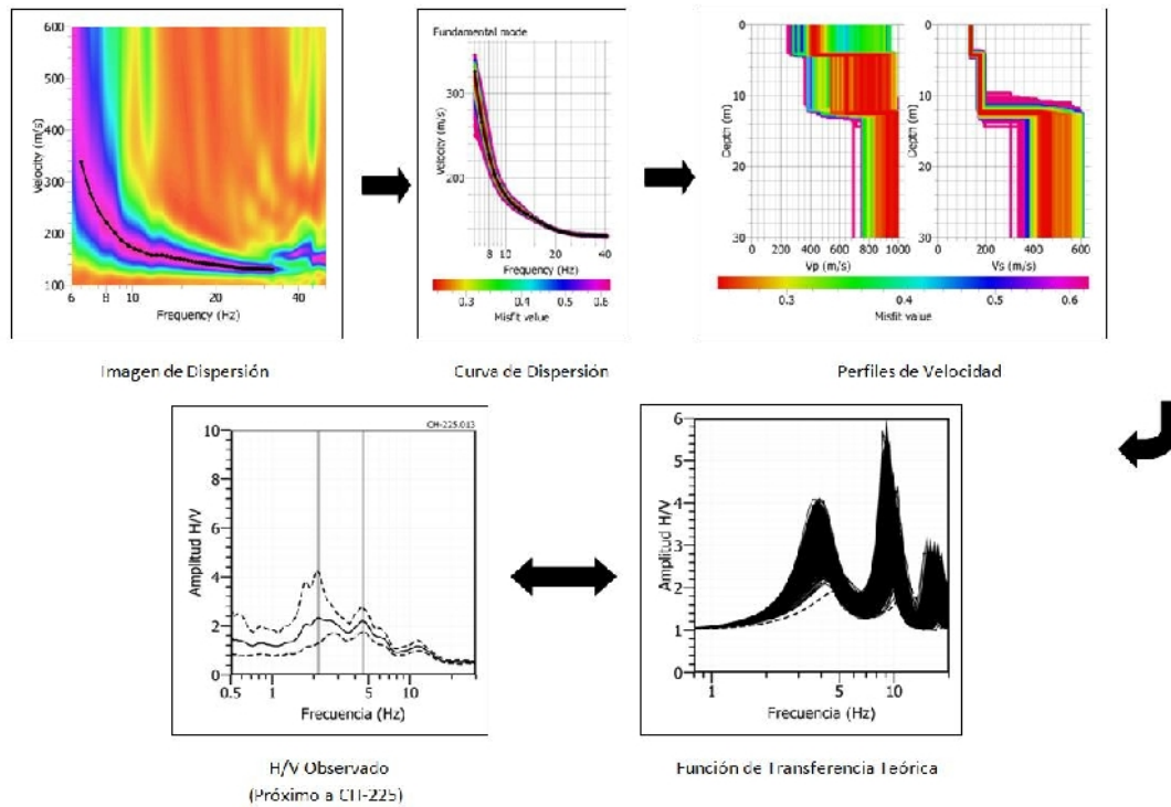
Figura 72b: Análisis e interpretación geofísica obtenida con el método MASW para el arreglo LR02-CH.
