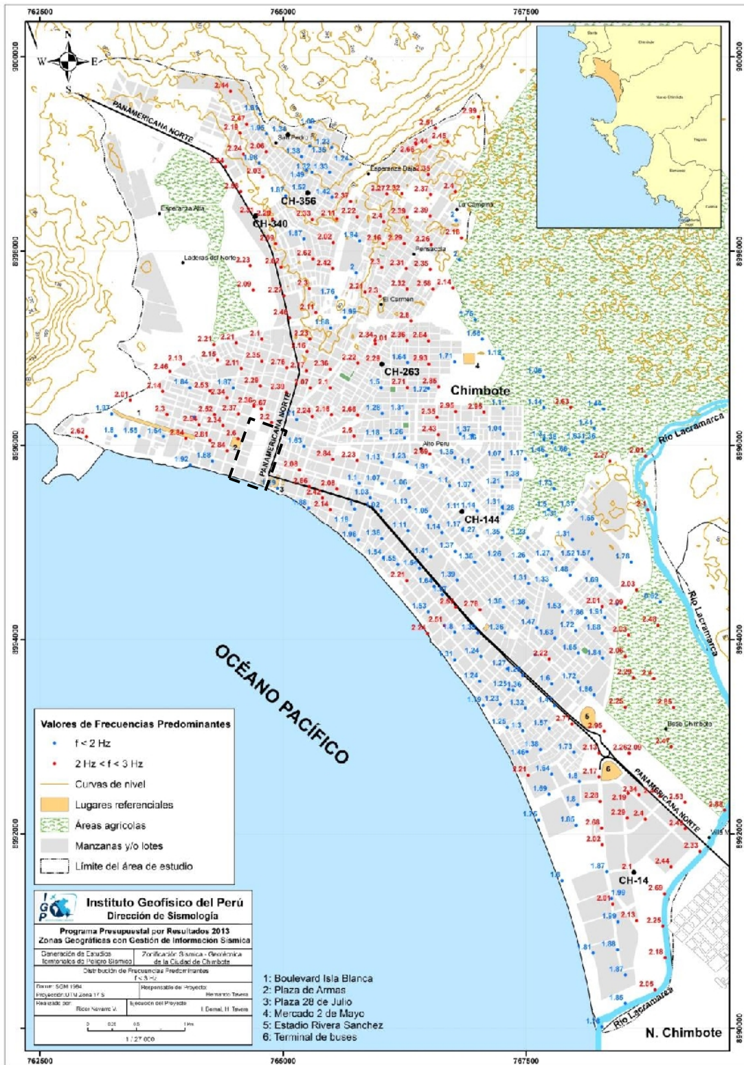
Figura 65: Mapa de la ciudad de Chimbote y distribución espacial de las frecuencias predominantes F_o ( F_p < 3.0 \text{ Hz} ). Los puntos en negro corresponden a ejemplos de H/V de la Figura 66. El recuadro indica la ubicación del área sin valores para F_o .
