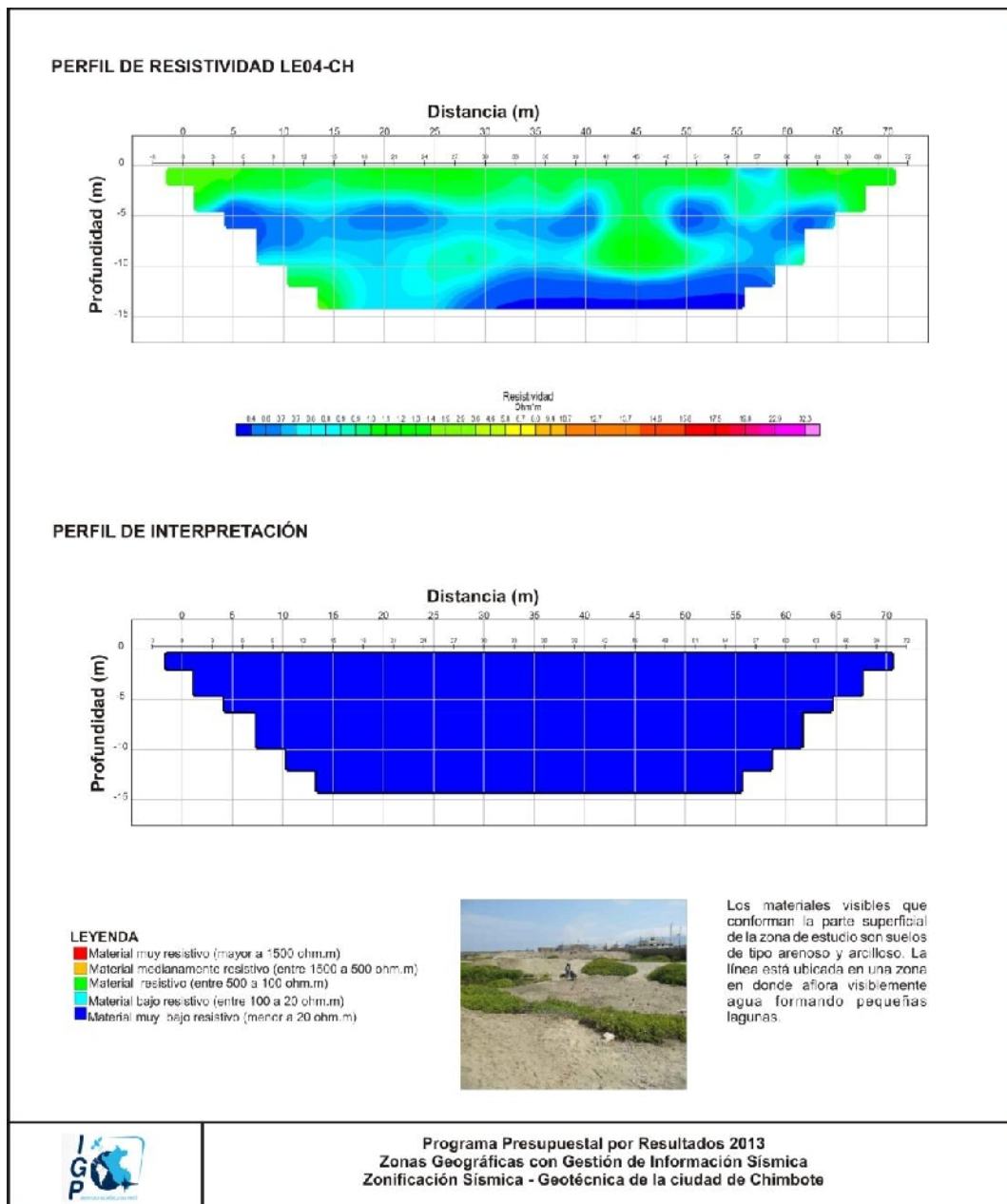
Figura 74d: Continuation.../ Línea de Tomografía Eléctrica LE04-CH tomada en el extremo sur de la ciudad de Chimbote y entre la línea de costa y el río Lacramarca.
