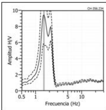
Figura 66: Ejemplos de razones espectrales (H/V) en el rango de frecuencias predominantes F_0 ( F_p < 3.0 Hz). Las líneas continuas representan la razón espectral y las discontinuas su desviación estándar. Las barras grises, definen la frecuencia predominante.
