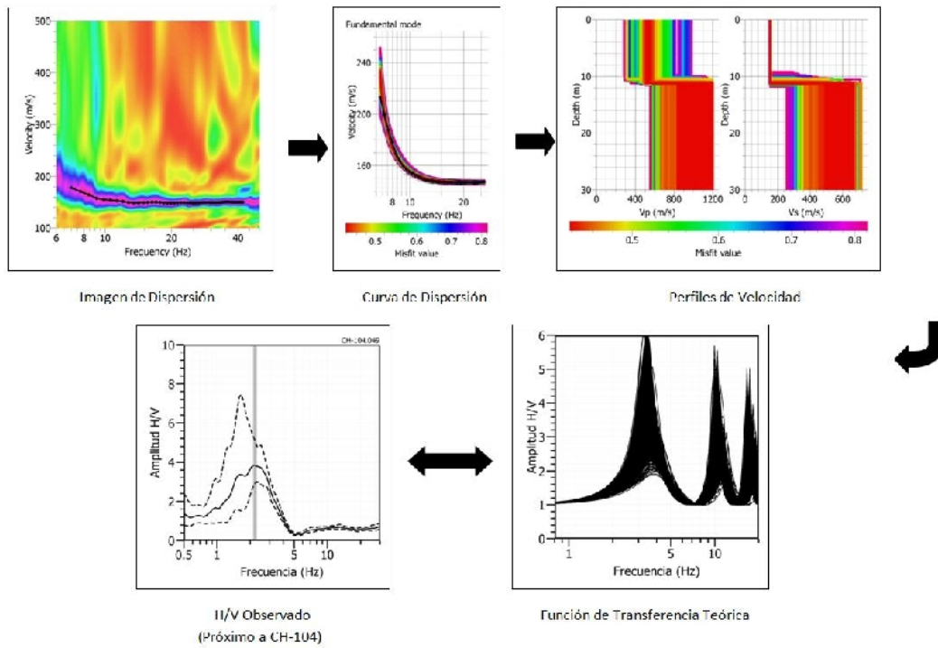
Figura 72c: Análisis e interpretación geofísica obtenida con el método MASW para el arreglo LR03-CH.
