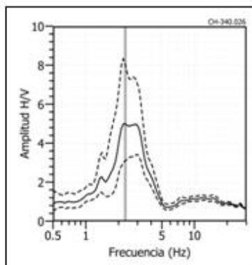
Figura 66: Continuación.../ Ejemplos de razones espectrales (H/V) obtenidos para puntos ubicados próximo a la línea de costa. Frecuencias predominantes F_0 ( F_p < 3.0 Hz).
