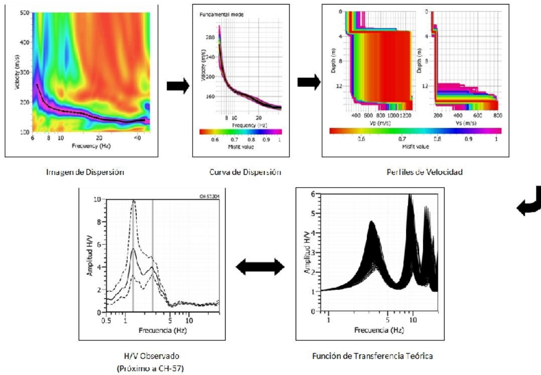
Figura 72d: Análisis e interpretación geofísica obtenida con el método MASW para el arreglo LR04-CH.
